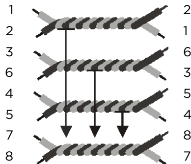
Ilustración 77 Efectos de 3 pares a 1 par
