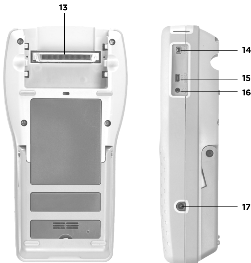
Ilustración 6 Terminal remoto (RH), vista trasera y lateral
