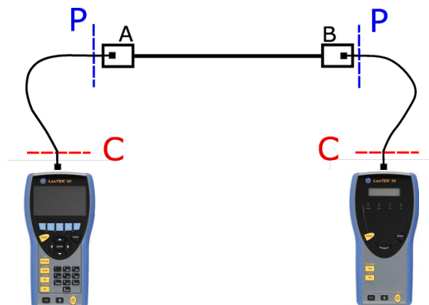
Ilustración 8 Estructura típica de comprobación
