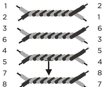
Ilustración 76 Efecto de par adyacente
